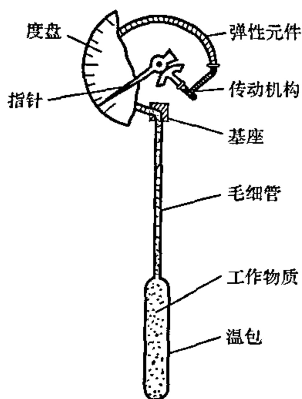
图 1 压力式温度计典型结构图
