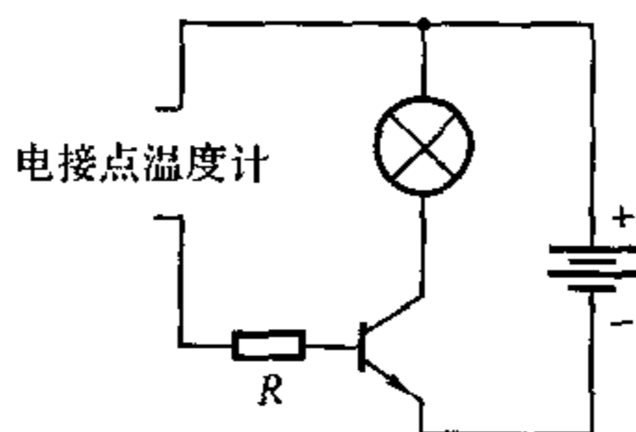
图2 信号电路
